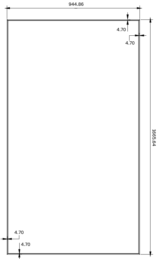
СХЕМА ДИСПЛЕЯ (ВИД СПЕРЕДИ)
